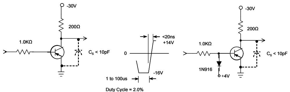
Fig. 1. Turn-On Time
